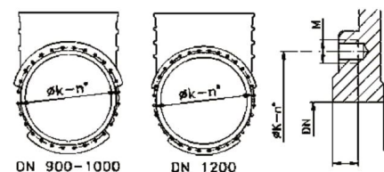
DN 900-1000
