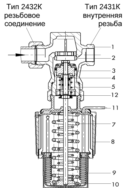
На рис. изображены: тип 2432 –слева и тип 2431K – справа Принцип действия обоих типов одинаков
