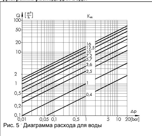
Диаграмма расхода для воды
