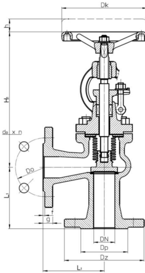
Вентиль сильфонний, фігура 235 F, I
